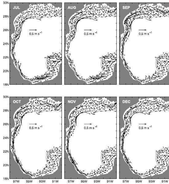
Figura 2.4: Corrientes superficiales promedio mensuales a lo largo del Golfo de México. Se muestran los datos correspondientes a los meses de julio a diciembre ([22]).
