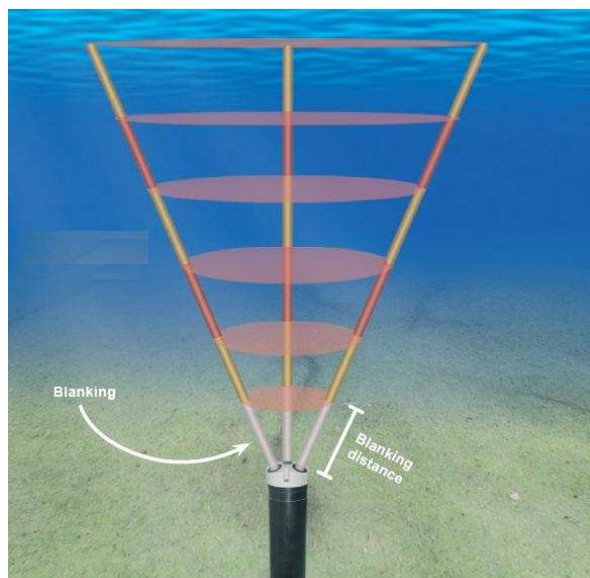
Figura 4.2: Ilustración de las celdas de un corrientímetro.
