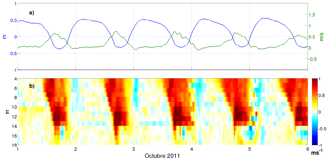
Figura 3.21: (a) Series de tiempo de elevación total (línea azul) y velocidad promediada en la vertical (línea verde) a lo largo del eje principal, y (b) perfil de corriente a lo largo del eje principal del 1 o al 6 de Octubre de 2011.
