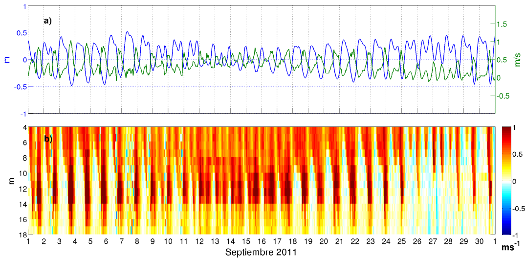
Figura 3.20: (a) Series de tiempo de elevación total (línea azul) y velocidad promediada en la vertical (línea verde) a lo largo del eje principal, y (b) perfil de corriente a lo largo del eje principal para el mes de Septiembre de 2011.
