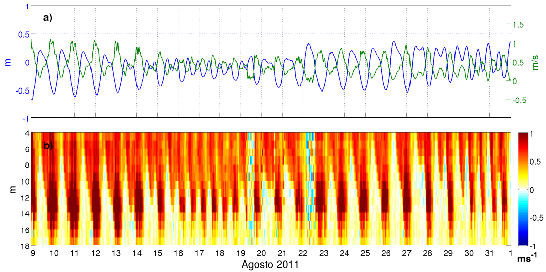
Figura 3.19: (a) Series de tiempo de elevación total (línea azul) y velocidad promediada en la vertical (línea verde) a lo largo del eje principal, y (b) perfil de corriente a lo largo del eje principal para el mes de Agosto de 2011.
