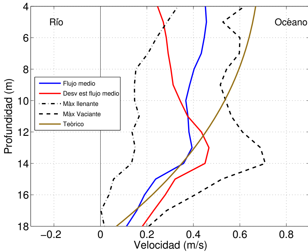
Figura 3.18: Flujo medio en la boca (línea azul) a lo largo del eje principal, desviación estándar del flujo medio (línea roja), flujo medio observado en la máxima llenante (puntos y líneas), flujo medio observado en la máxima vaciante (línea punteada) y perfil teórico (línea café).
