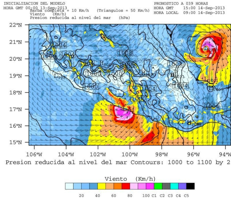
Figura 2.7: Dominio 2 del pronóstico operativo del grupo Interacción Oceano-Atmósfera.
