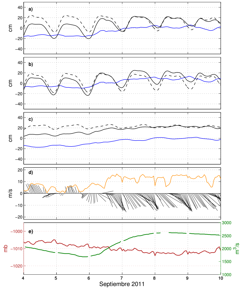
Figura 3.11: La elevación total (línea negra continua), la marea pronosticada (línea negra punteada) y el residual armónico (línea azul), para los sitios de a) la laguna Tlalixcoyan, b) la Boca de la laguna Tlalixcoyan, y c) el río Limón, durante el evento del 6 al 10 de Septiembre de 2011. d) la rapidez (línea anaranjada) y dirección del viento (astillas negras) a 10 metros arriba de la superficie, e) la presión atmosférica multiplicada por -1 (línea roja) y el gasto del río (línea verde).
