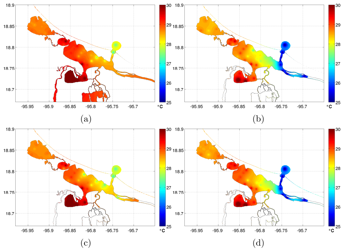
Figura 3.27: (a) Temperatura máxima, (b) temperatura mínima, (c) temperatura en superficie y (d) temperatura en fondo para la campaña 4 (18-20 de Marzo, 2012).
