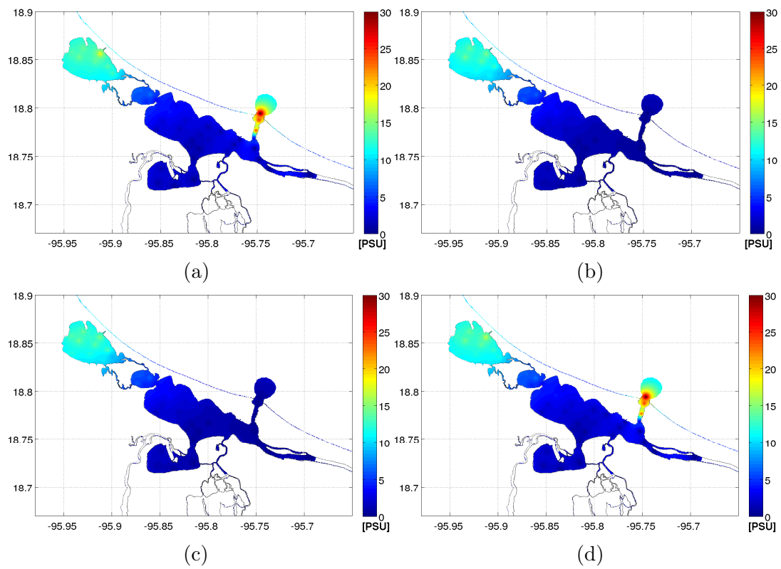
Figura 3.22: (a) Salinidad máxima, (b) salinidad mínima, (c) salinidad en superficie y (d) salinidad en fondo para la campaña 2 (1º y 2 de Agosto, 2011).
