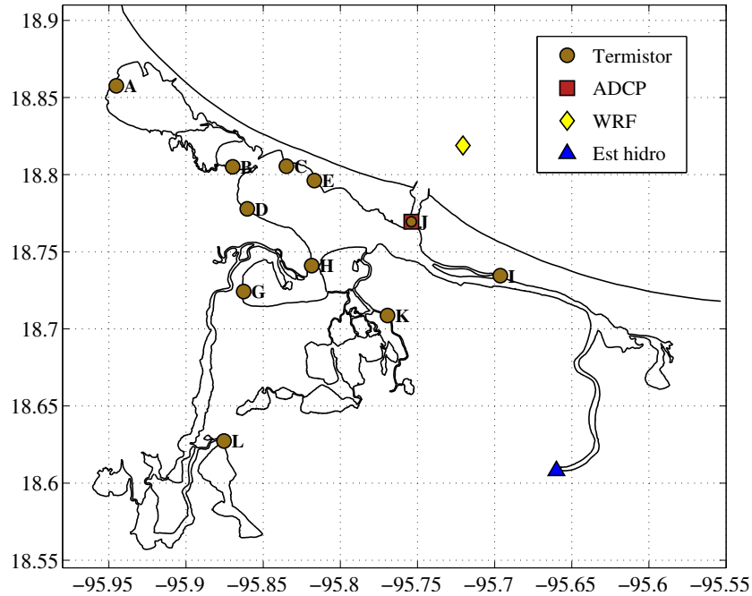
Figura 2.1: Ubicación de los sensores de presión y temperatura (círculos), el corrientímetro (cuadrado), el punto de malla donde se extrajo información meteorológica (diamante) y la estación hidrométrica de la CONAGUA (triángulo).
