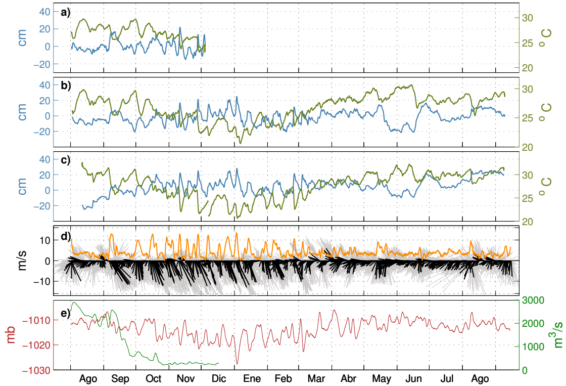
Figura 3.6: El residual filtrado (línea azul) y la temperatura observada (línea verde olivo) filtrada con medias móviles de 26 hrs, para los sitios de a) la Boca; b) el río Papaloapan; y c) el río Acula, para los años 2011-2012. d) la rapidez (línea anaranjada) y dirección del viento en astillas (sin filtrar grises, filtradas negras) a 10 metros arriba de la superficie, e) la presión atmosférica multiplicada por -1 (línea roja) y el gasto del río Papaloapan (línea verde), también se muestran.
