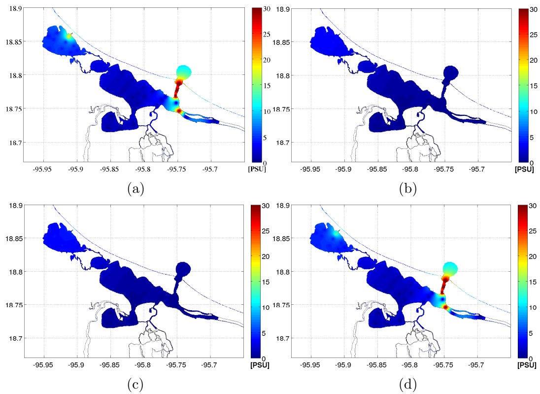
Figura 3.30: (a) Salinidad máxima, (b) salinidad mínima, (c) salinidad en superficie y (d) salinidad en fondo para la campaña 6 (9 y 10 de Septiembre, 2012).
