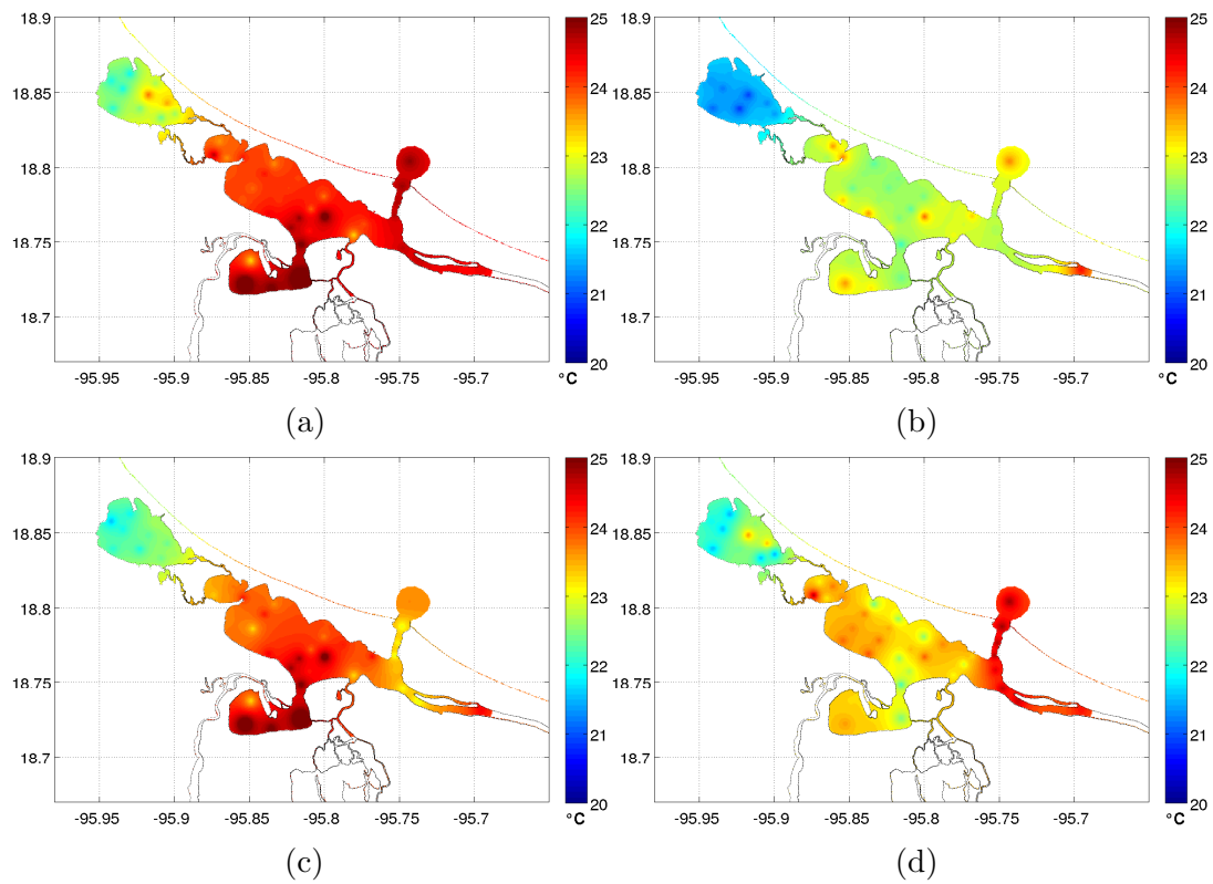
Figura 3.25: (a) Temperatura máxima, (b) temperatura mínima, (c) temperatura en superficie y (d) temperatura en fondo para la campaña 3 (3 y 5 de Diciembre, 2011).
