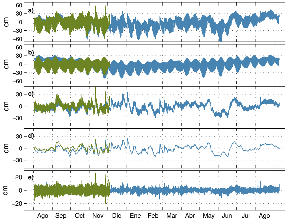
Figura 3.1: Componentes que forman la a) elevación total: b) marea pronosticada y c) residual armónico; y los componentes que forman el residual armónico: d) el residual inducido por procesos, obtenido por filtrado; y e) el residual causado por interacción de procesos, obtenido al substrair el residual filtrado del residual armónico en los sitios de la Boca (línea verde olivo) y el río Papaloapan (línea azul) para los años 2011-2012. La escala de los ejes varía para que los residuales puedan identificarse con claridad. Los sitios estan indicados en la figura 2.1.
