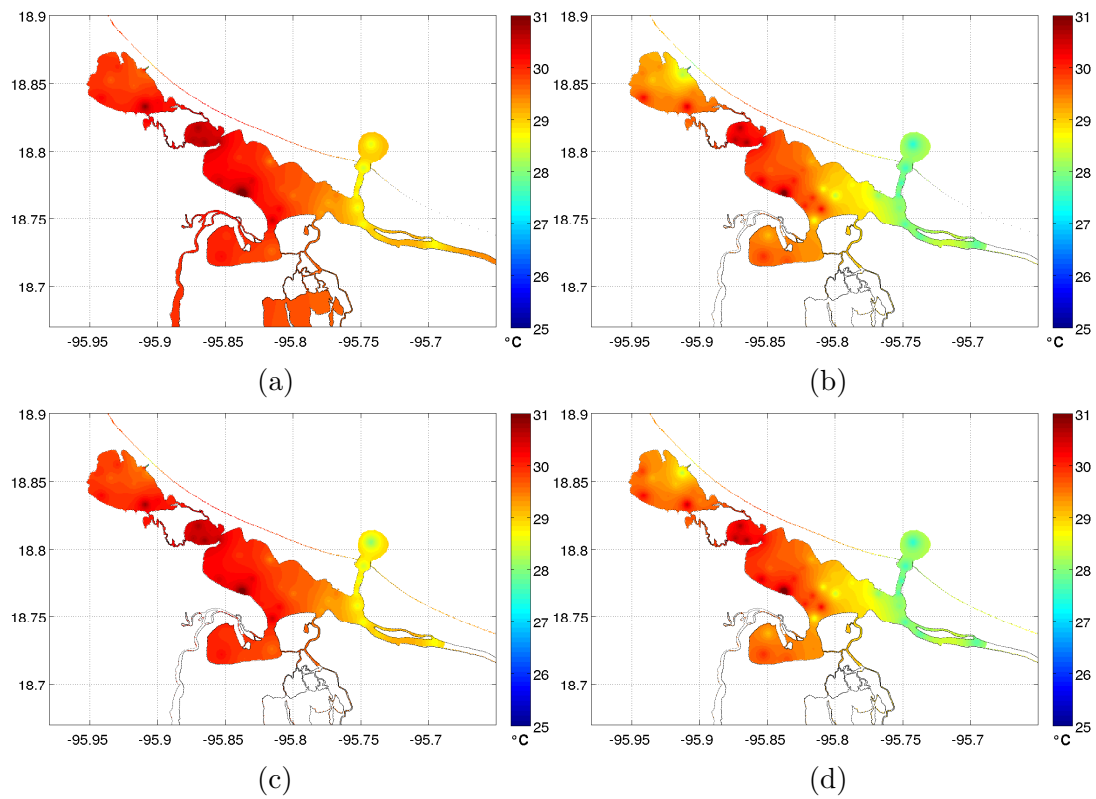
Figura 3.29: (a) Temperatura máxima, (b) temperatura mínima, (c) temperatura en superficie y (d) temperatura en fondo para la campaña 5 (19 y 20 de Mayo, 2012).
