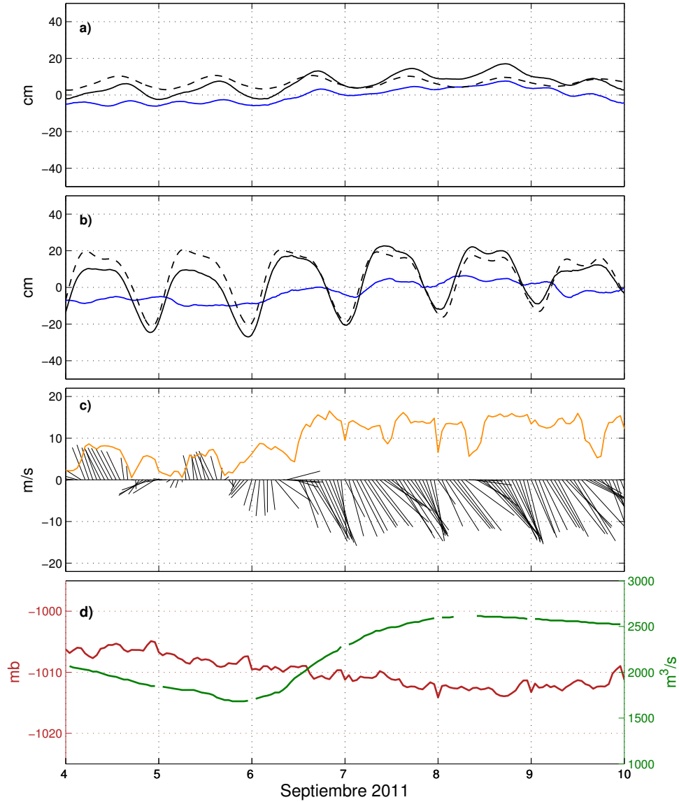
Figura 3.12: La elevación total (línea negra continua), la marea pronosticada (línea negra punteada) y el residual armónico (línea azul), para los sitios de a) la laguna Camaronera, y b) la laguna Buen País), durante el evento del 6 al 10 de Septiembre de 2011. c) la rapidez (línea anaranjada) y dirección del viento (astillas negras) a 10 metros arriba de la superficie, d) la presión atmosférica invertida (línea roja) y el gasto del río (línea verde).
