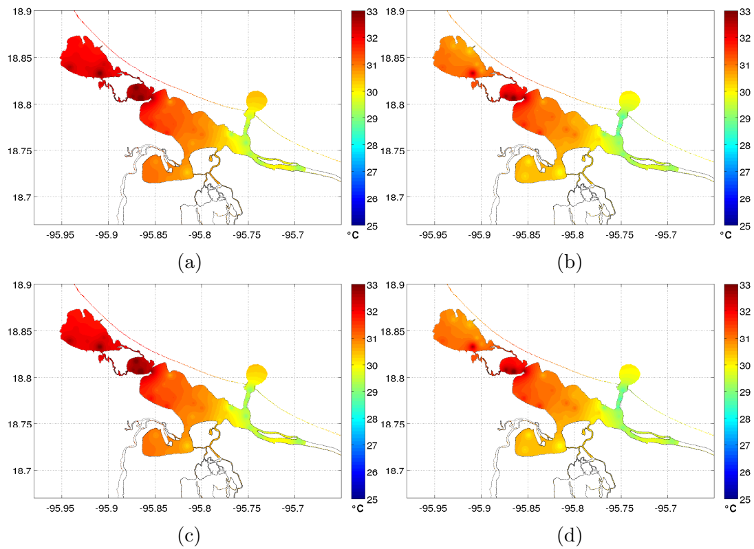
Figura 3.31: (a) Temperatura máxima, (b) temperatura mínima, (c) temperatura en superficie y (d) temperatura en fondo para la campaña 6 (9 y 10 de Septiembre, 2012).
