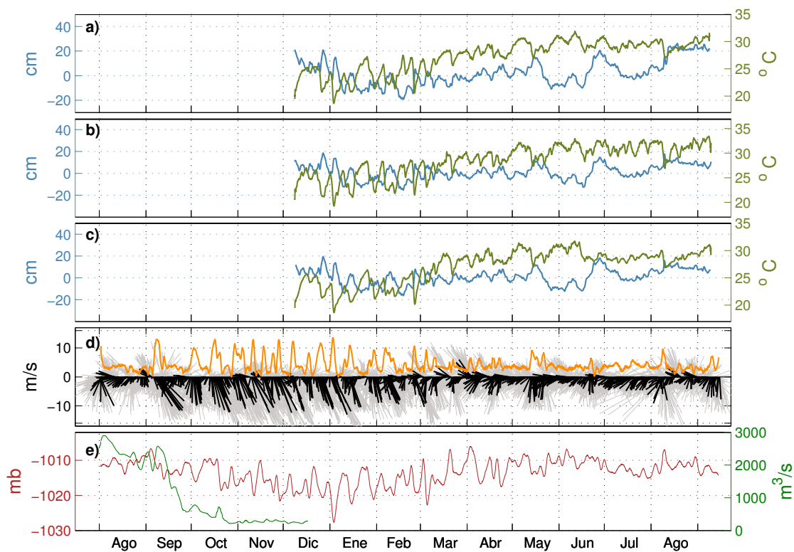
Figura 3.8: El residual filtrado (línea azul) y la temperatura observada (línea verde olivo) filtrada con medias móviles de 26 hrs, para los sitios de a) la laguna de Alvarado 1; b) la laguna de Alvarado 2; y c) la laguna de Alvarado 3, para los años 2011-2012. d) la rapidez (línea anaranjada) y dirección del viento en astillas (sin filtrar grises, filtradas negras) a 10 metros arriba de la superficie, e) la presión atmosférica multiplicada por -1 (línea roja) y el gasto del río (línea verde), también se muestran.
