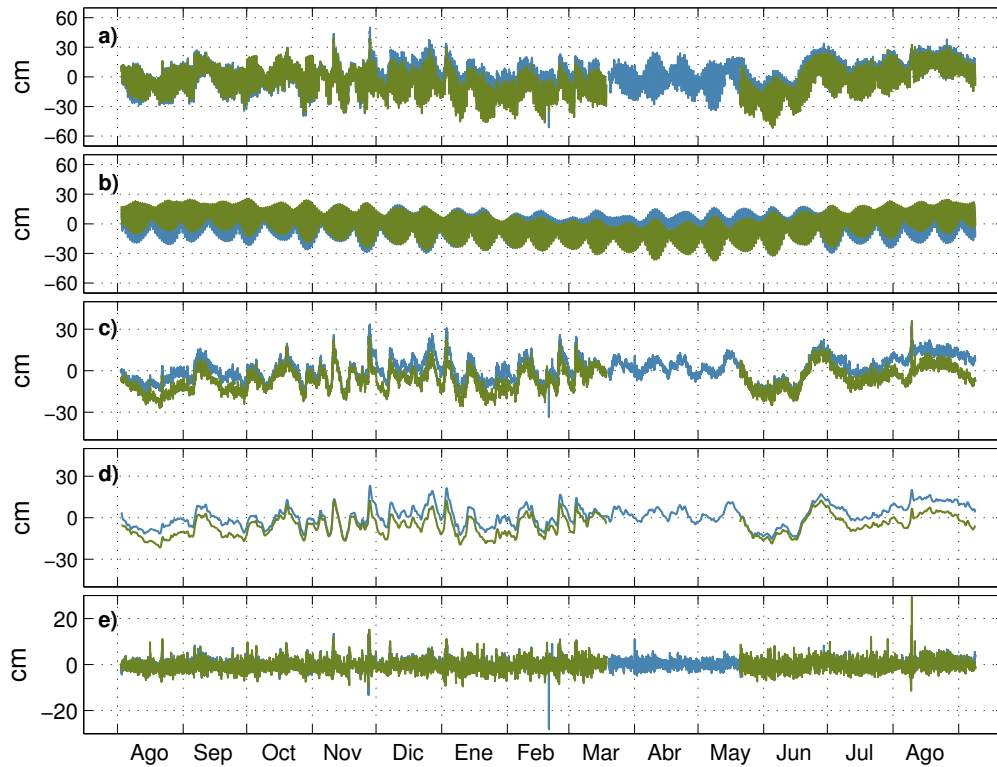
Figura 3.5: Componentes que forman la a elevación total): b) marea pronosticada y c) residual armónico; y los componentes que forman el residual armónico: d) el residual inducido por procesos, obtenido por filtrado; y e) el residual causado por interacción de procesos, obtenido al substrar el residual filtrado del residual armónico en los sitios de la laguna de Tlalixcoyan (línea verde olivo) y la boca de la laguna de Tlalixcoyan (línea azul) para los años 2011-2012. Loa escala de los ejes varía para que los residuales puedan identificarse con claridad. Los sitios estan indicados en la figura 2.1.
