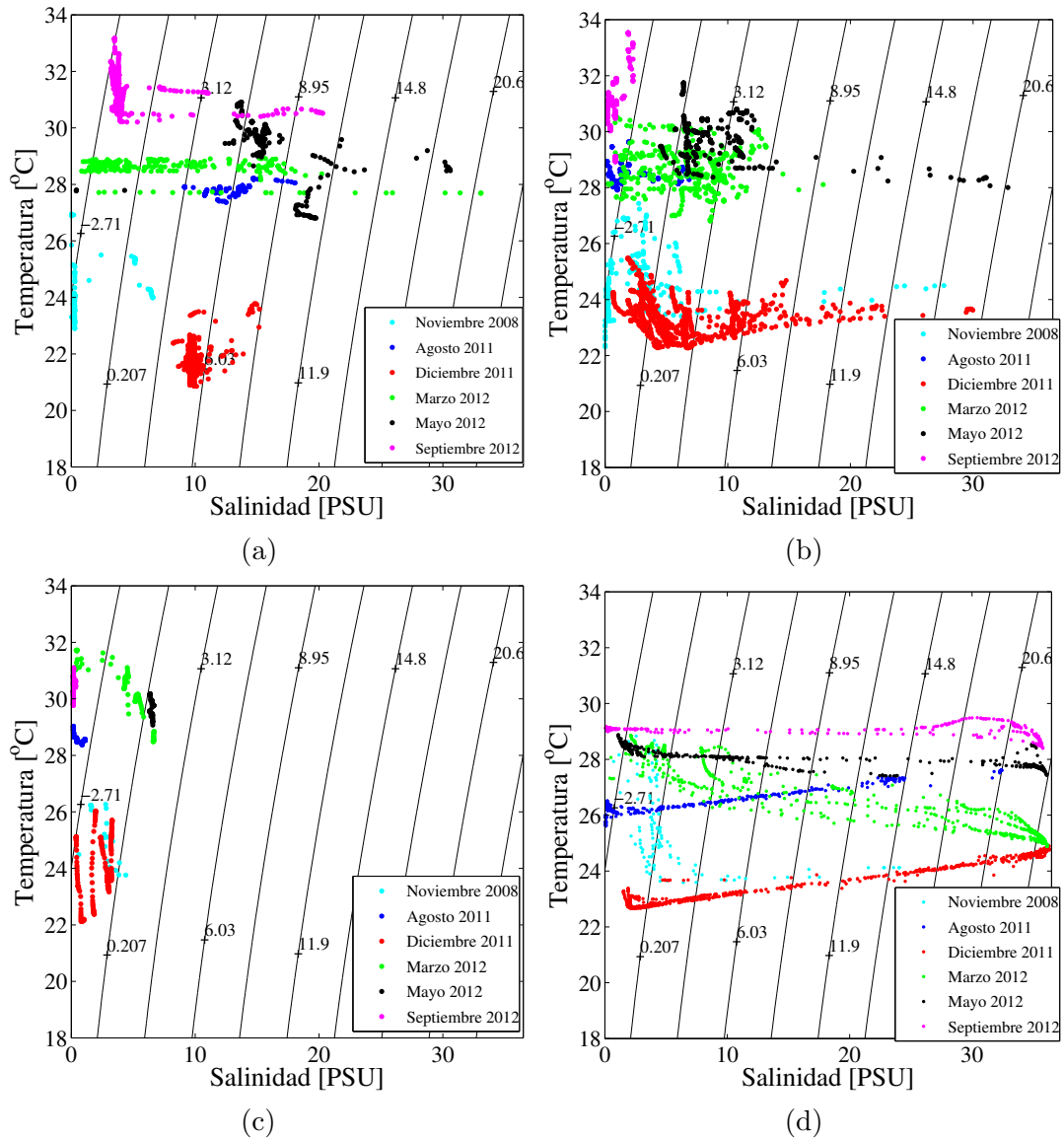
Figura 3.34: Diagramas T-S para la Zona 1 (laguna Camaronera) (a), Zona 2 (lagunas de Alvarado y Buen País) (b), Zona 3 (laguna Tlalixcoyan) (c) y Zona 4 (Río Papaloapan y la Boca) (d).
