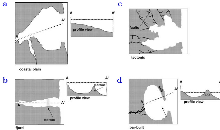
Figura 1.2: Tipos de estuarios en base a su geomorfología: a) planicie costera, b) fiordo, c) tectónico y d) hecho por barrera. Figura tomada de Valle-Levinson (2010) [22].
