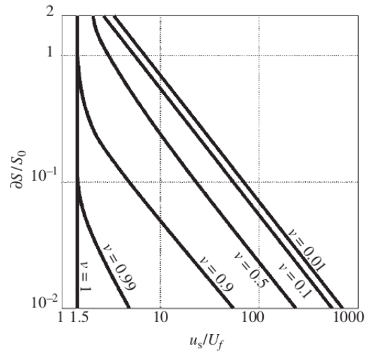
Figura 1.4: Fracción de flujo de sal difusiva en el espacio del parámetro de estratificación/circulación. El transporte de sal esta dominado por procesos advectivos bajo una alta circulación gravitacional o condiciones de estratificación fuertes, X y por procesos difusivos cuando el parámetro de circulación es bajo independientemente del parámetro de estratificación. Figura tomada de Valle-Levinson (2010) [22].
