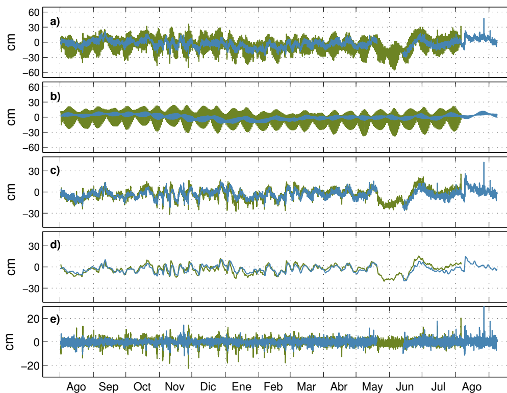
Figura 3.4: Componentes que forman la a) elevación total: b) marea pronosticada y c) residual armónico; y los componentes que forman el residual armónico: el residual d) inducido por procesos, obtenido por filtrado; y el e) residual causado por interacción de procesos, obtenido al substrar el residual armónico - residual filtrado en los sitios de la laguna Camaronera (línea azul) y la laguna Buen País (línea verde olivo) para los años 2011-2012. La escala de los ejes varía para que los residuales puedan identificarse con claridad. Los sitios están indicados en la figura 2.1.
