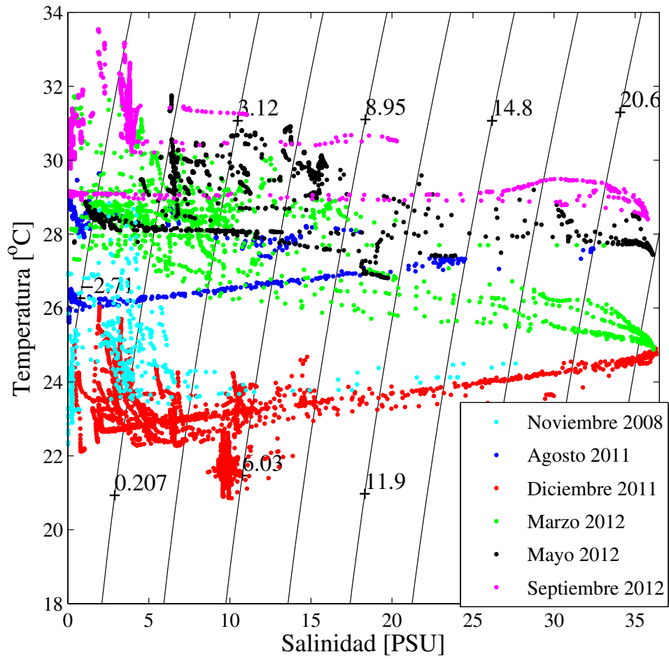
Figura 3.32: Diagrama T-S de todas las campañas de medición.
