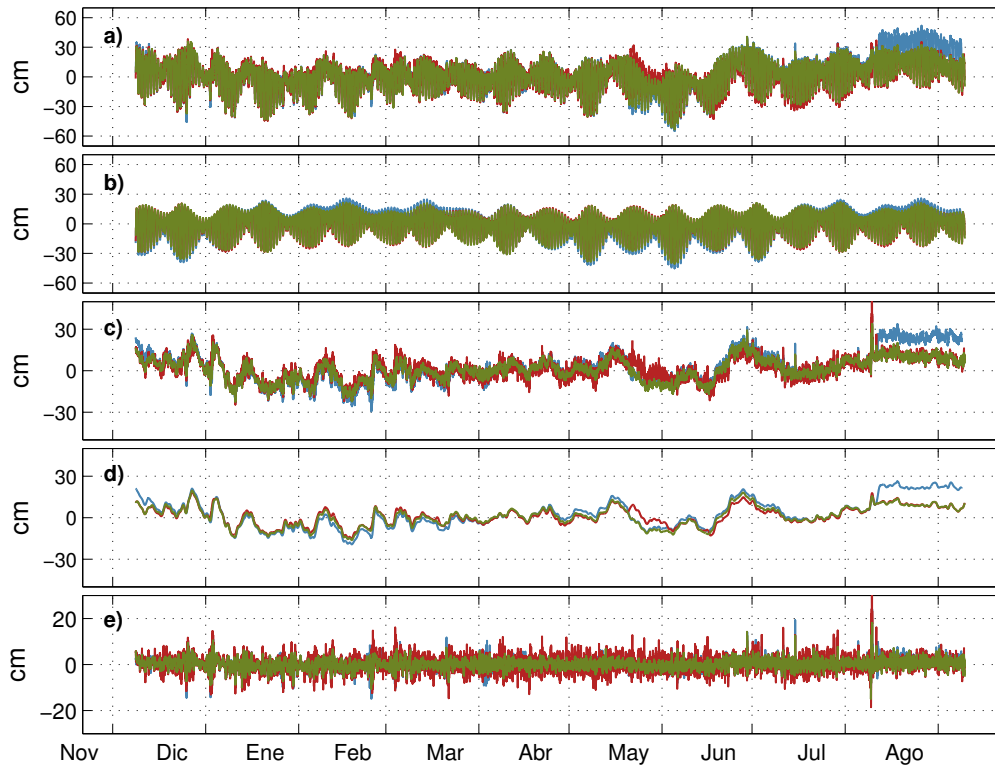
Figura 3.2: Componentes que forman la a) elevación total: b) marea pronosticada y c) residual armónico; y los componentes que forman el residual armónico: d) el residual inducido por procesos, obtenido por filtrado; y e) el residual causado por interacción de procesos, obtenido al substrair el residual filtrado del residual armónico en los sitios de la laguna de Alvarado 1 (línea azul) Alvarado 2 (línea roja) Alvarado 3 (línea verde olivo) para los años 2011-2012. La escala de los ejes varía para que los residuales puedan identificarse con claridad. Los sitios están indicados en la figura 2.1.
