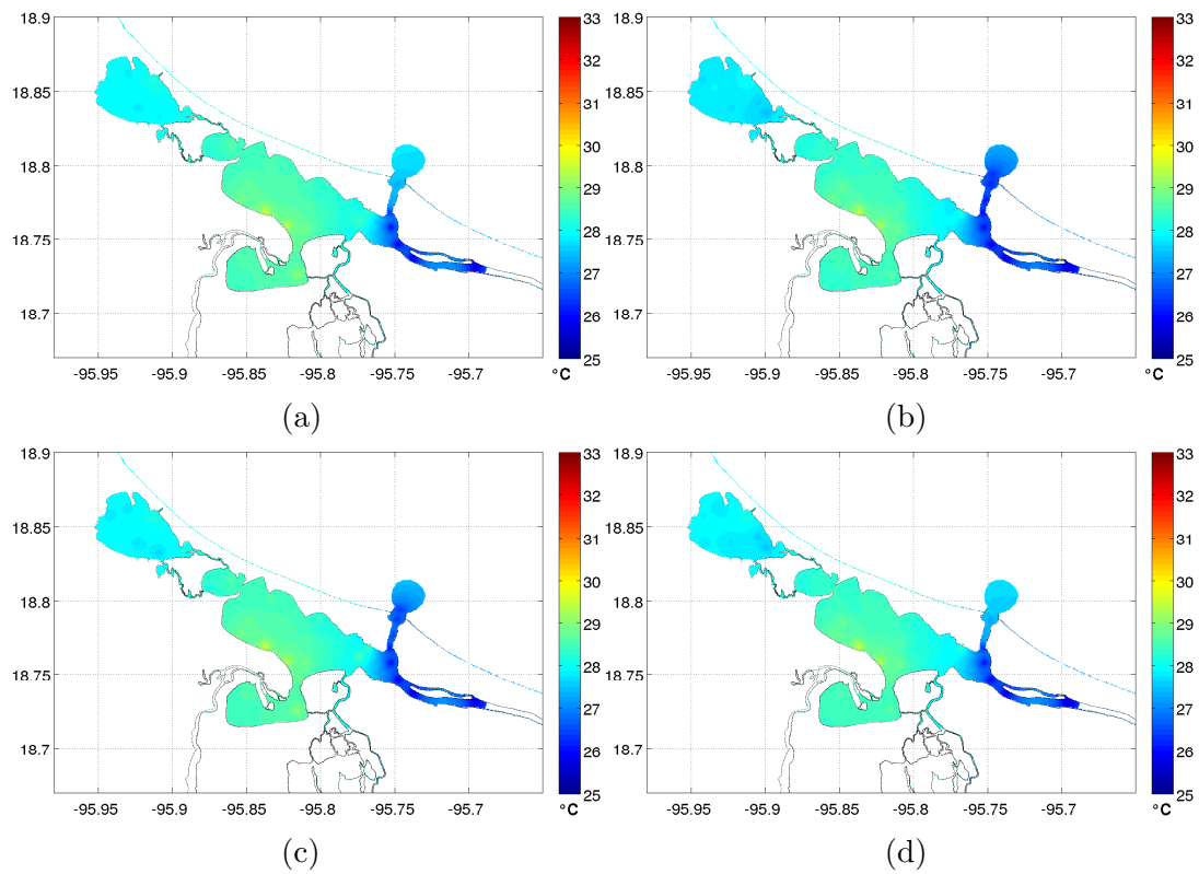
Figura 3.23: (a) Temperatura máxima, (b) temperatura mínima, (c) temperatura en superficie y (d) temperatura en fondo para la campaña 2 (1 o y 2 de Agosto, 2011).
