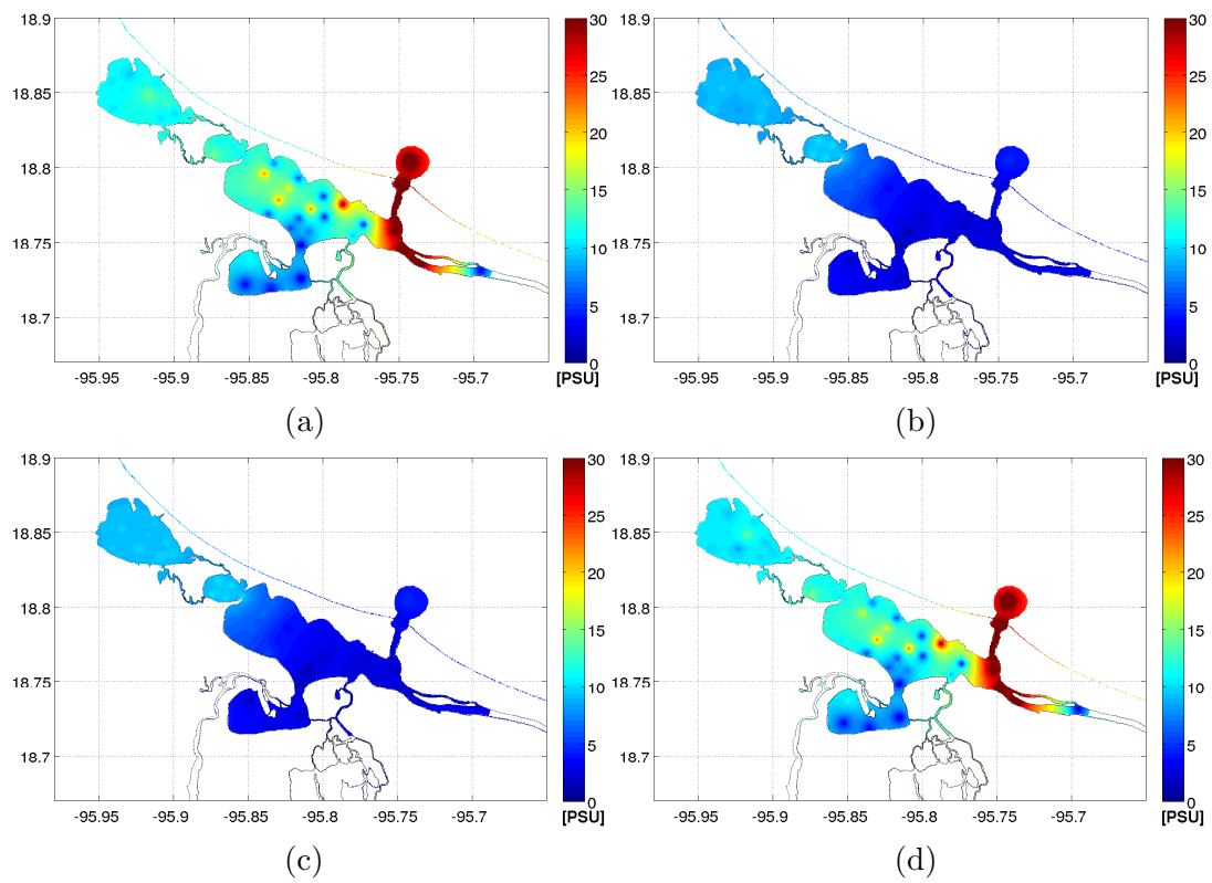
Figura 3.24: (a) Salinidad máxima, (b) salinidad mínima, (c) salinidad en superficie y (d) salinidad en fondo para la campaña 3 (3 y 5 de Diciembre, 2011).
