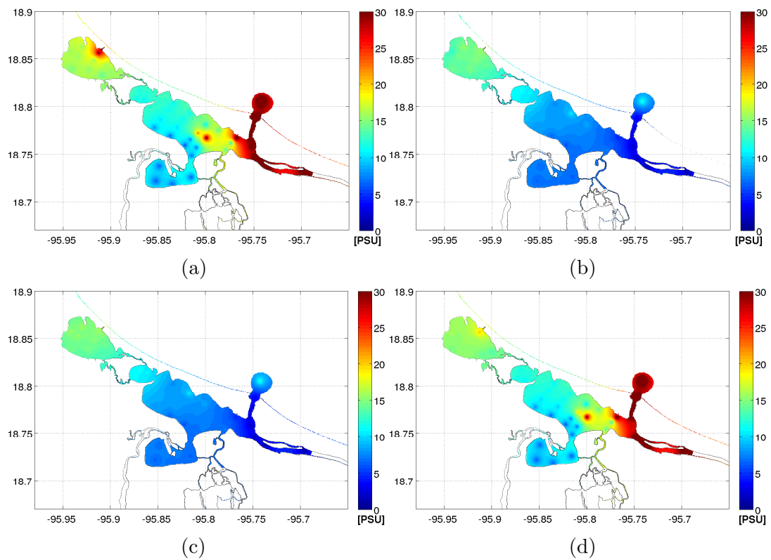
Figura 3.28: (a) Salinidad máxima, (b) salinidad mínima, (c) salinidad en superficie y (d) salinidad en fondo para la campaña 5 (19 y 20 de Mayo, 2012).
