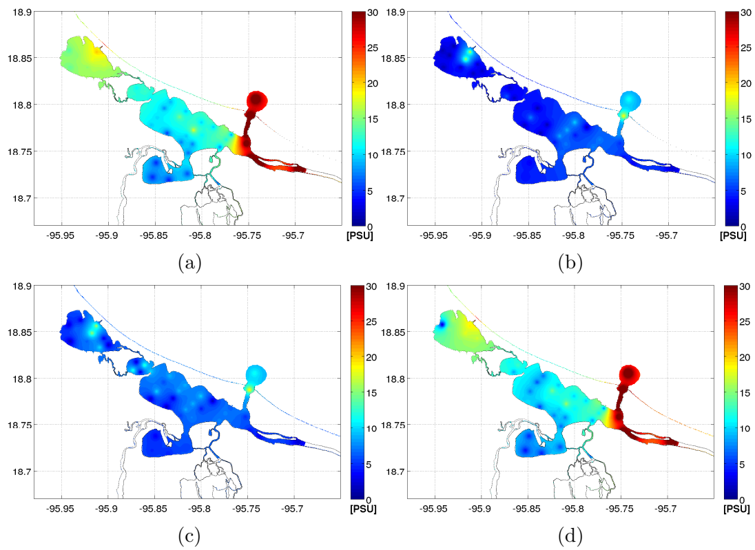
Figura 3.26: (a) Salinidad máxima, (b) salinidad mínima, (c) salinidad en superficie y (d) salinidad en fondo para la campaña 4 (18-20 de Marzo, 2012).
