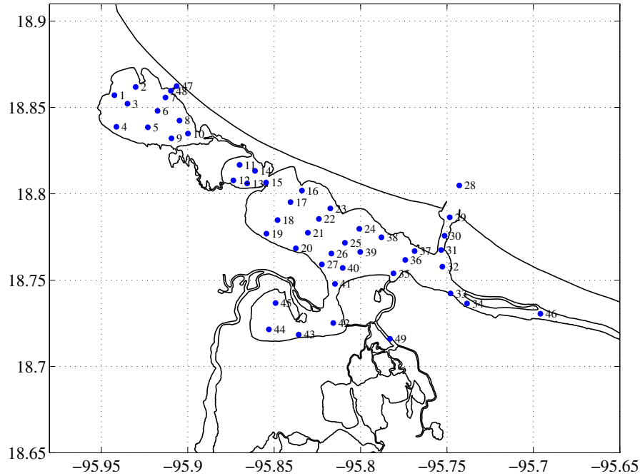
Figura 2.6: Red de estaciones de CTD.
