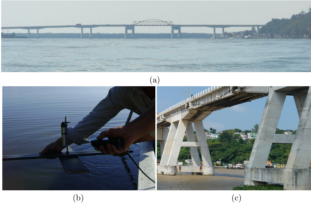
Figura 2.3: (a) Puente Alvarado visto desde adentro de la laguna, (b) cruceta con sensor de presión y (c) pilar del puente Alvarado donde se colocó el ADCP.
